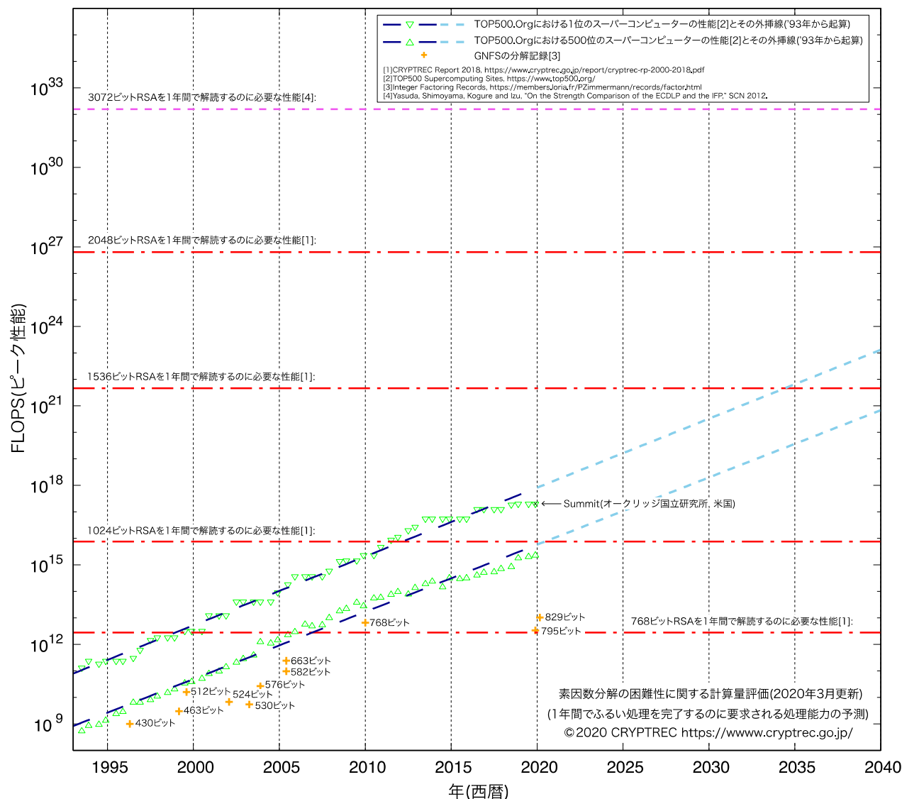
図 3.1：素因数分解の困難性に関する計算量評価
