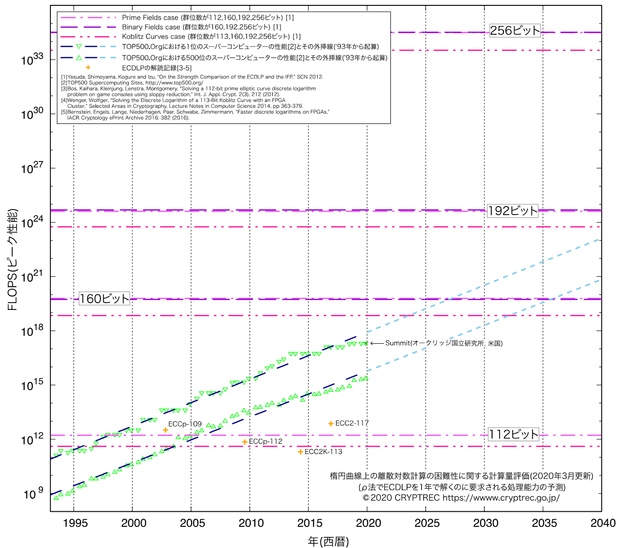
図 3. 2 : 楕円曲線上の離散対数計算の困難性に関する計算量評価 ( \rho 法でECDLPを1年で解くのに要求される処理能力の予測、2020年3月更新) 4
