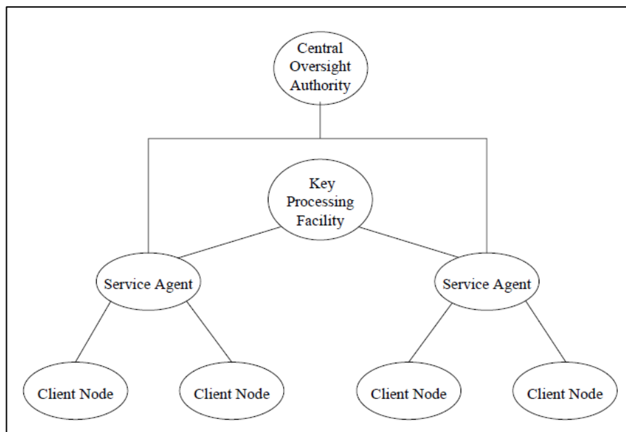
図 1.3.2 鍵管理の基盤 (KMI) の概念
