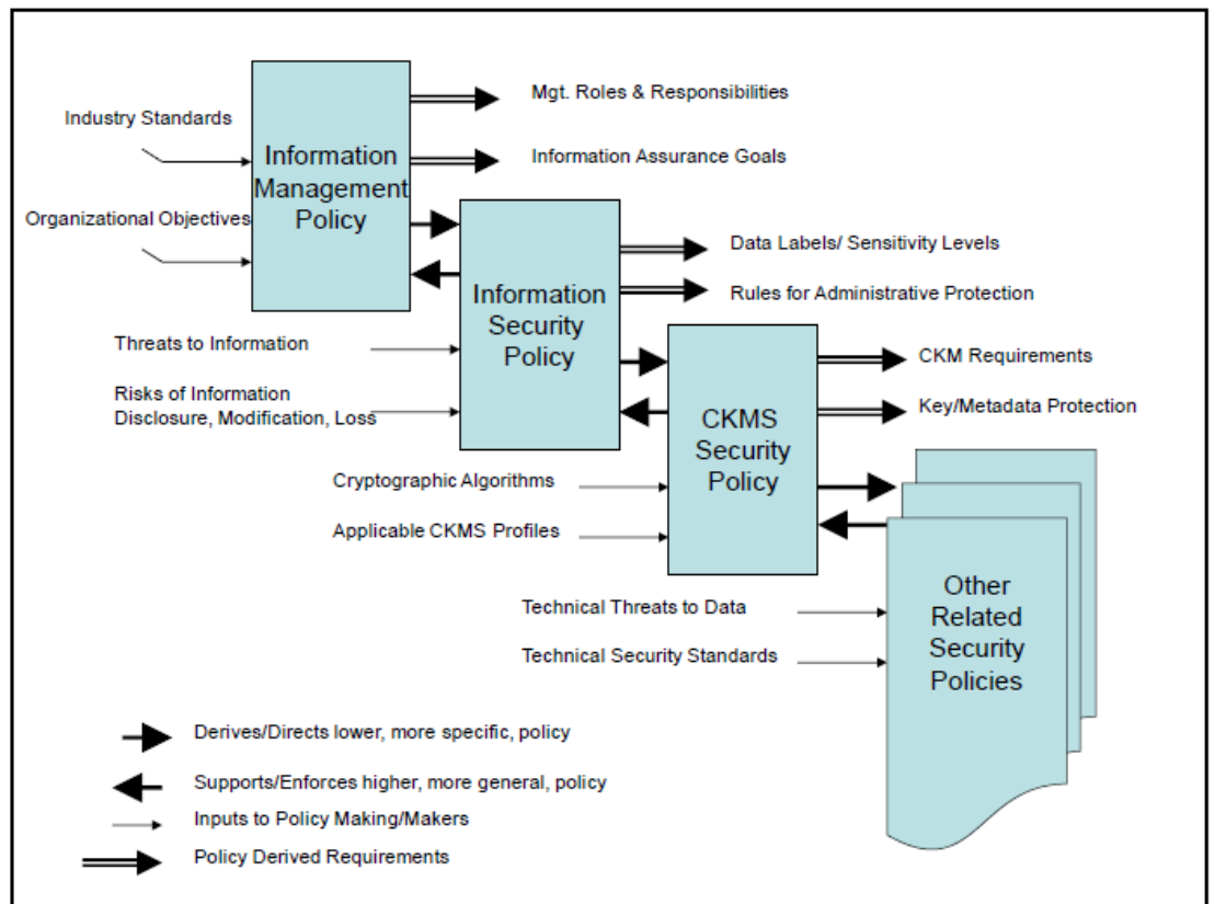
図 1.3.3 セキュリティポリシーの関連図
